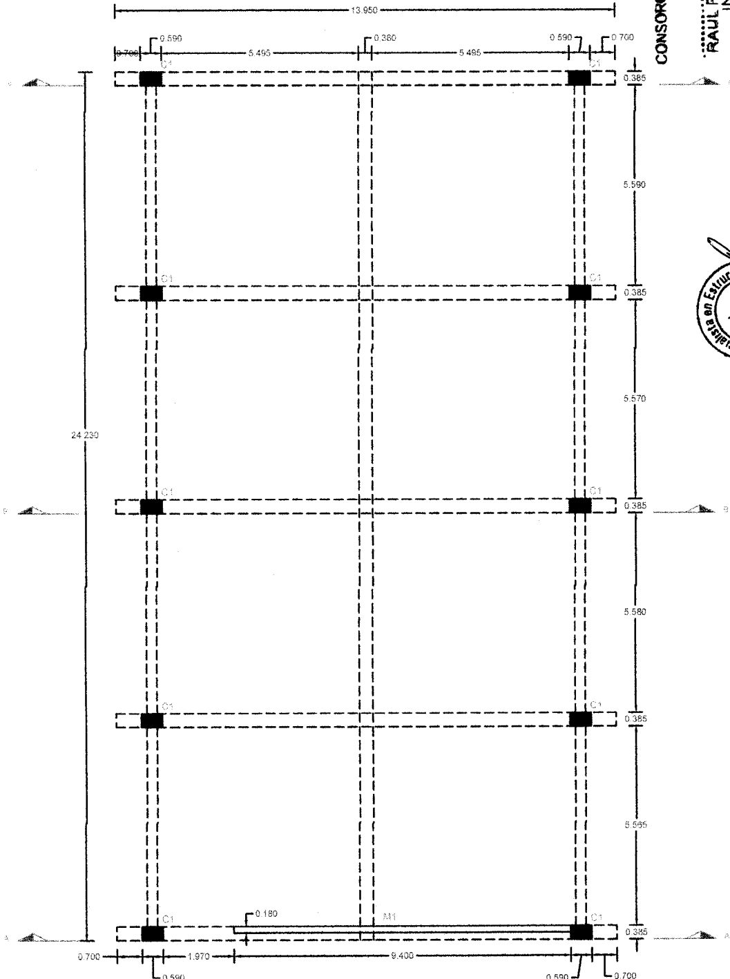
PLANTA PISO 1
